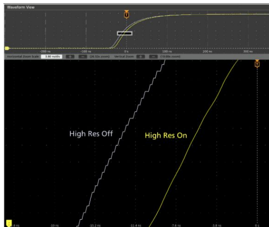
5 系列 MSO 的 12 位 ADC 与全新 High Res 模式相结合, 实现了业界领先的垂直分辨率。
